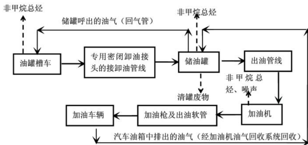
图 5-2 本项目营运期工艺流程
