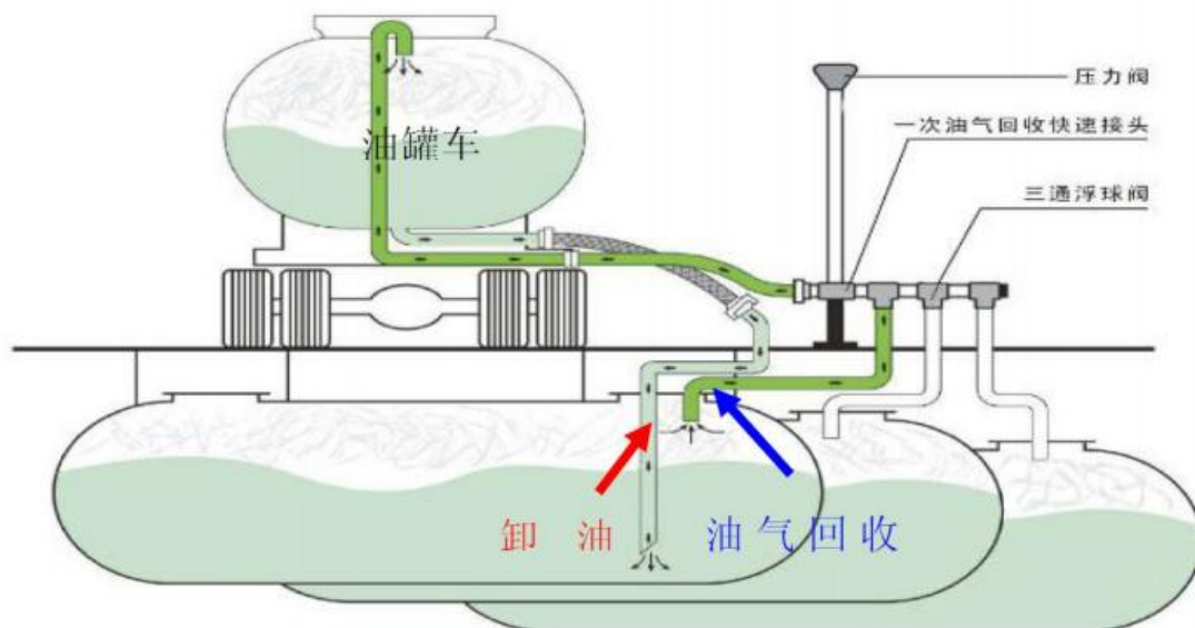
图 5-3 第一次油气回收系统示意图
