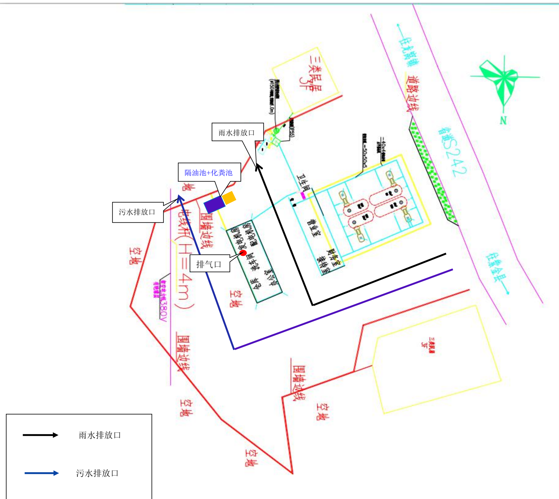
附图3 项目平面布置图
